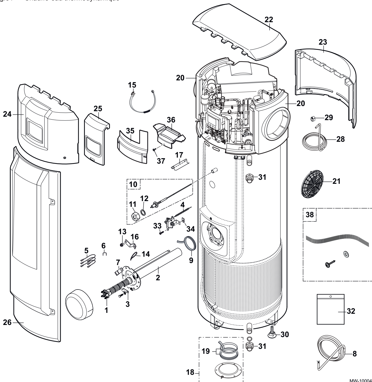
Fig.51 Chauffe-eau thermodynamique
